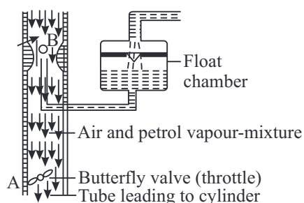
Fig. 9.36: Carburettor
